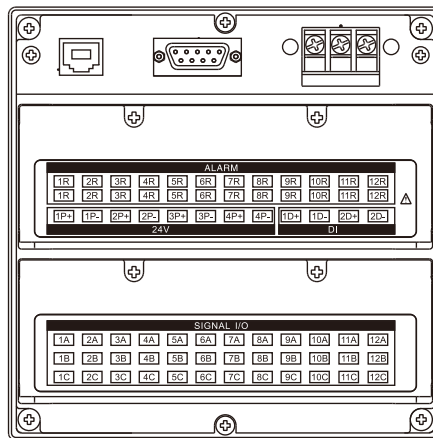
MS6316端子排列
