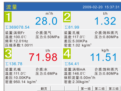
-流量显示-
